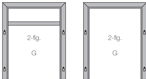
Zweiflügelige Zarge, geschosshoch
